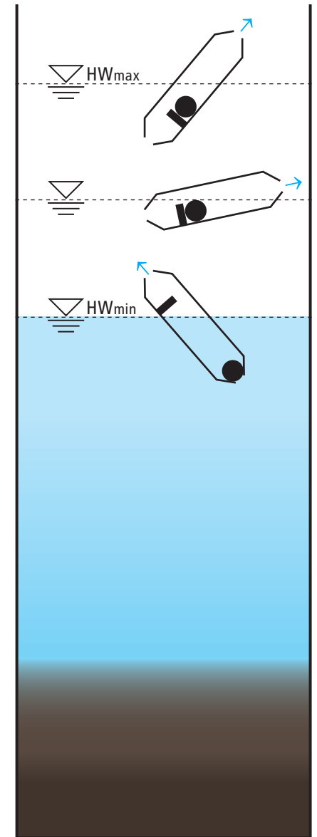
Heberspülung und Klarwasserabzug
